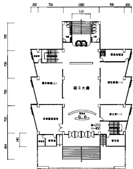
山岳博物館一樓平面圖
