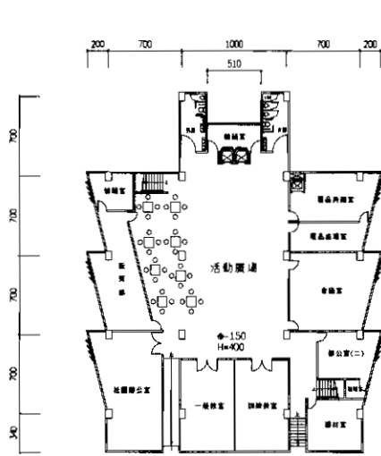
山岳博物館地下一樓平面圖
